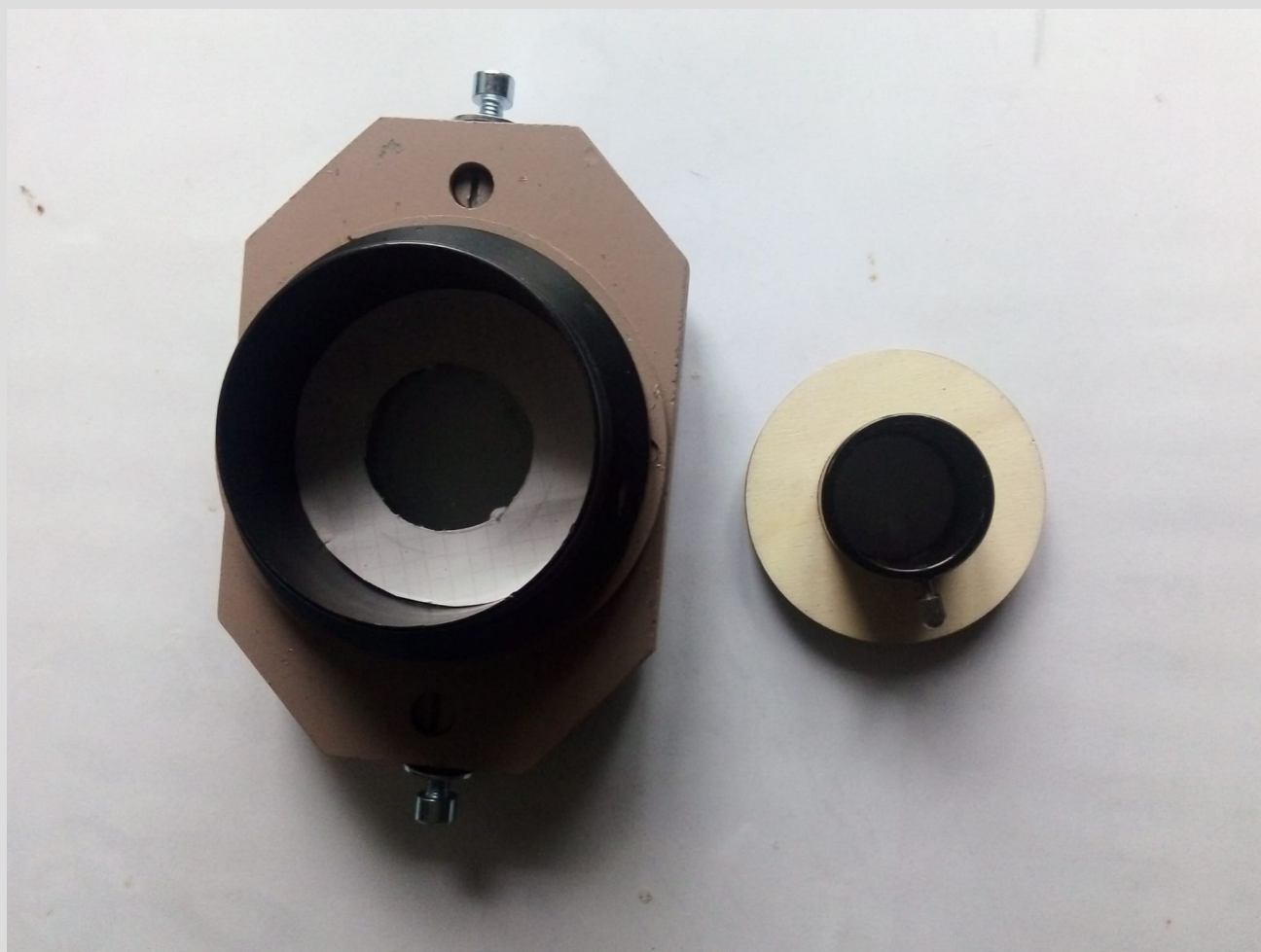
Porte objectif + support laser pour réglages
