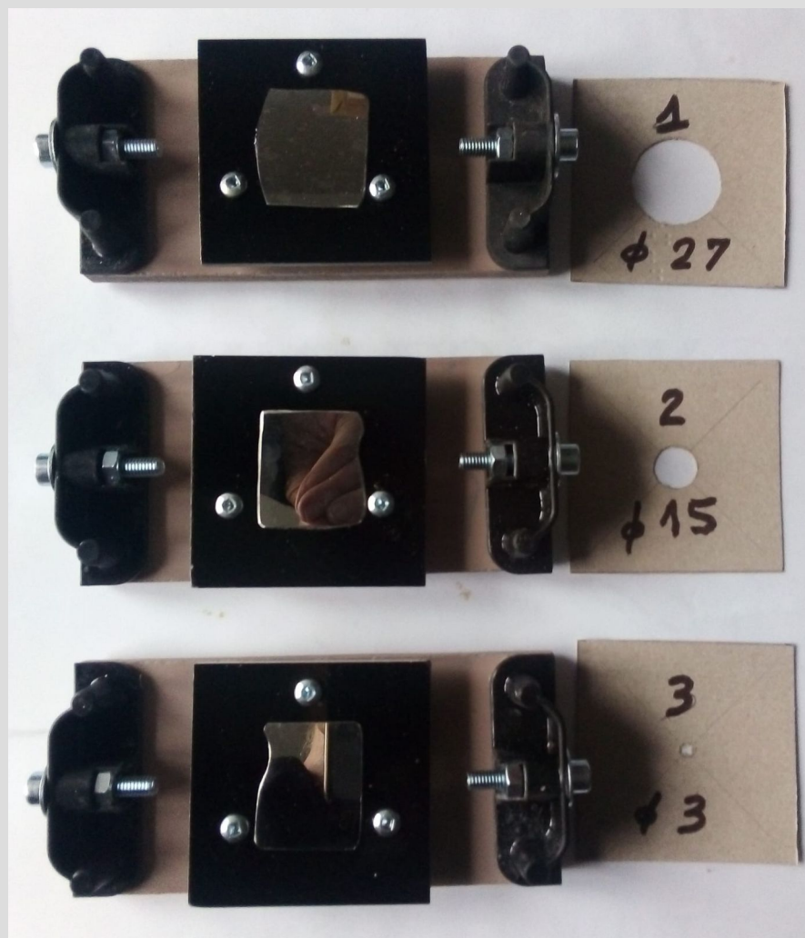
Supports miroirs + simulateurs largeur faisceaux
